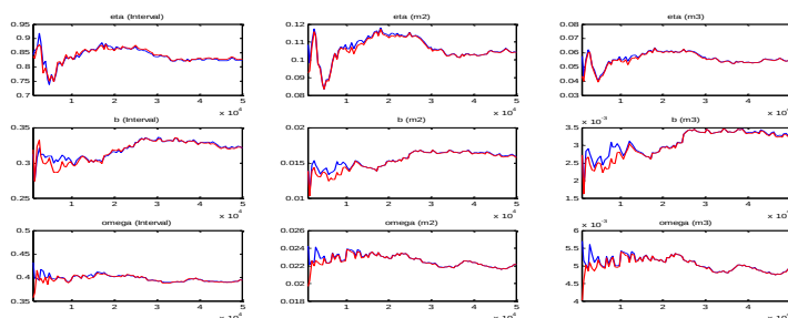
نمودار ۱. MCMC
