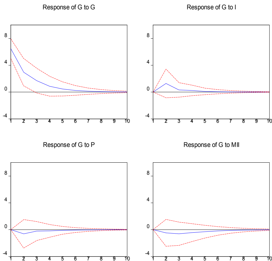
نمودار ۲. توابع عکس‌العمل آنی (ضربه و واکنش)
