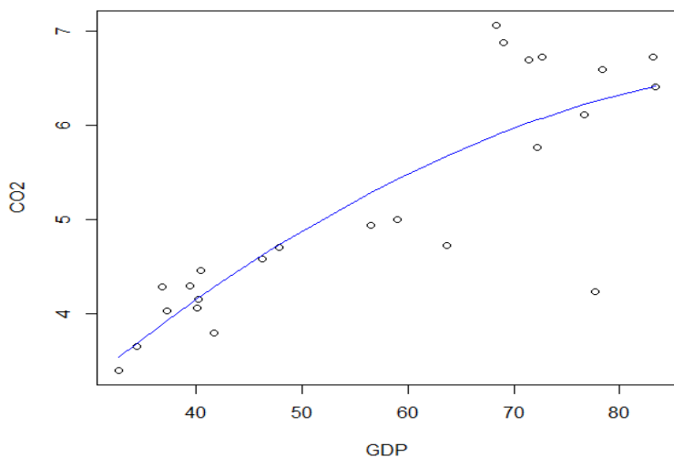
نمودار ۳. برازش ناپارامتریک رابطه \text{CO}_2 و GDP با روش P-Spline (با استفاده از داده‌های ایران)
