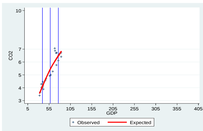
نمودار ۲. برازش ناپارامتریک رابطه \text{CO}_2 و GDP با روش RC Spline (با استفاده از داده‌های ایران)
