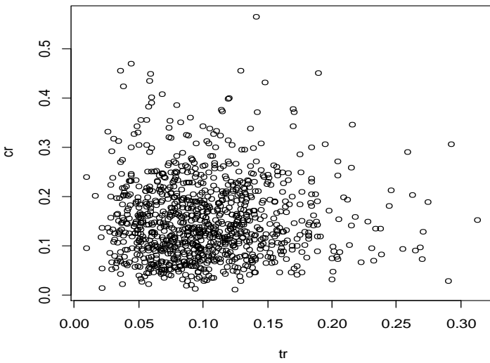
شکل ۳. نمایی از تابع توزیع مشترک استخراج شده
