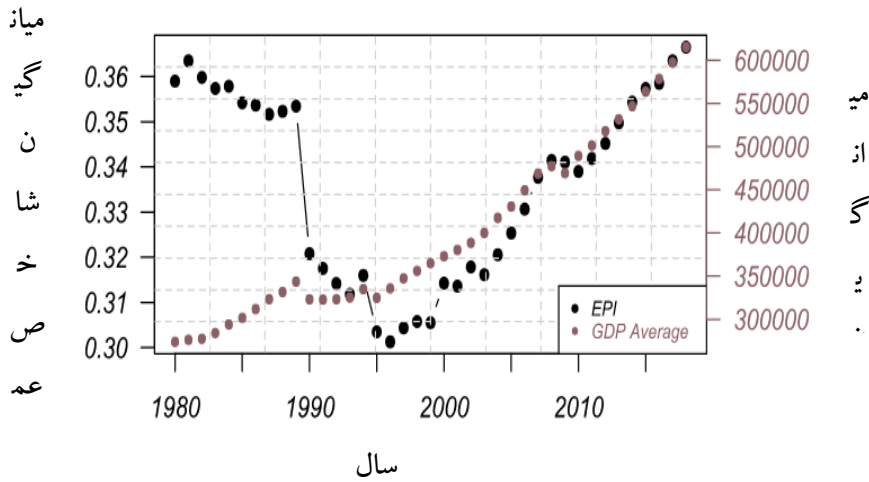
نمودار ۲. مقایسه روند میانگین شاخص عملکرد محیط زیست و درآمد سرانه
