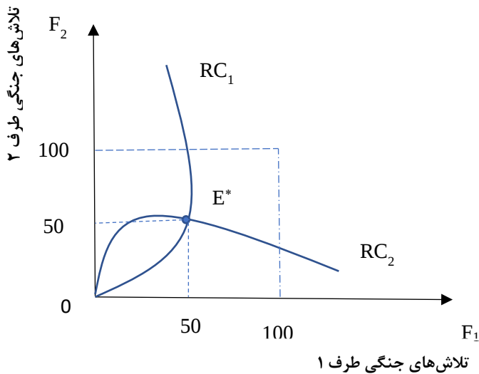
شکل ۱. منحنی‌های واکنش در یک مدل درگیری
