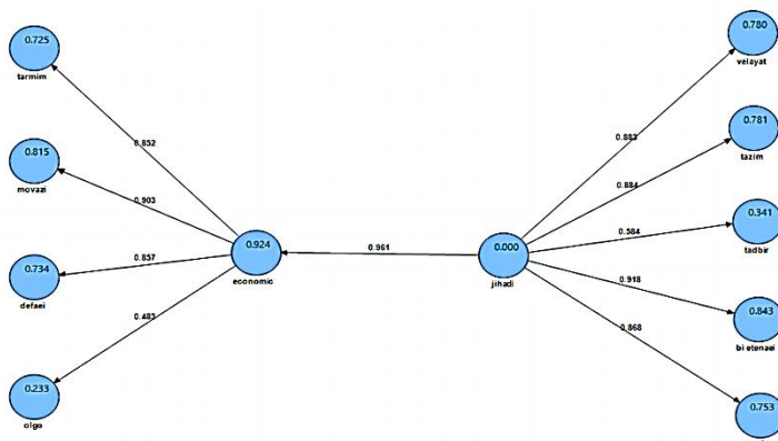
شکل ۴. ضریب مسیر
