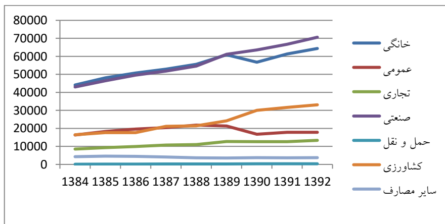
نمودار ۱. روند مصرف انرژی الکتریکی به تفکیک بخش‌های مصرفی طی سال‌های ۱۳۸۴-۱۳۹۲ (گیگاوات ساعت)
