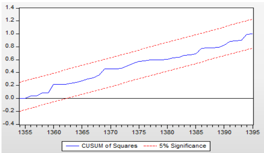
شکل ۹. نمودار CUSUMSQ برای مدل (۱۸)
